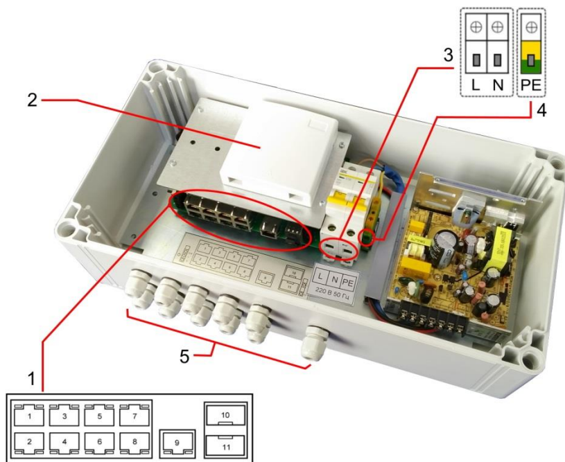
Рис.4 Подключение коммутатора SW-60812/W
