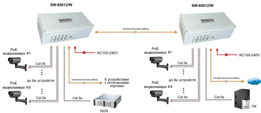
Рис.7 Схема каскадного подключения коммутатора SW-60812/W
