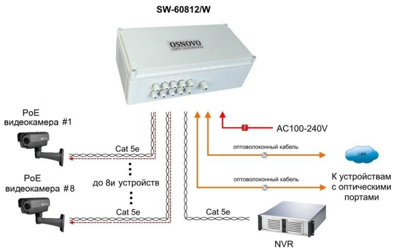
Рис.6 Типовая схема подключения коммутатора SW-60812/W
