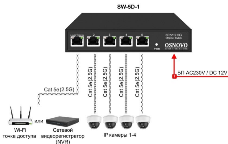
Рис.4 Типовая схема подключения коммутатора SW-5D-1
