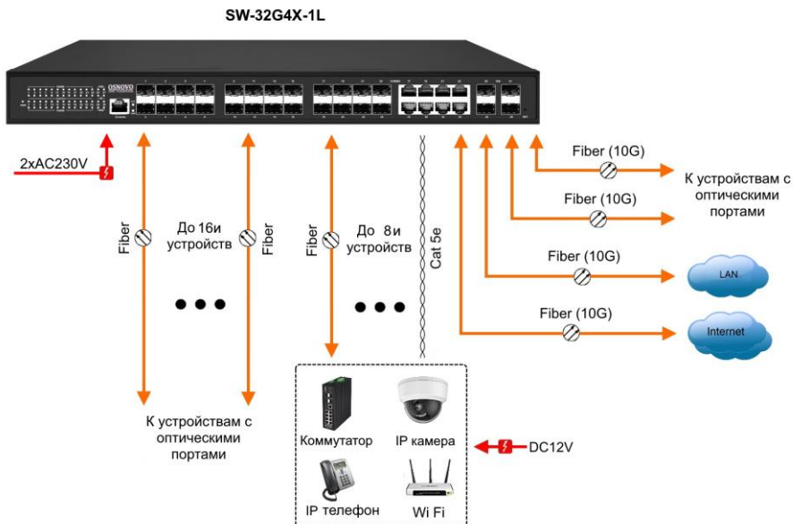
Рис.5 Типовая схема подключения коммутатора SW-32G4X-1L
