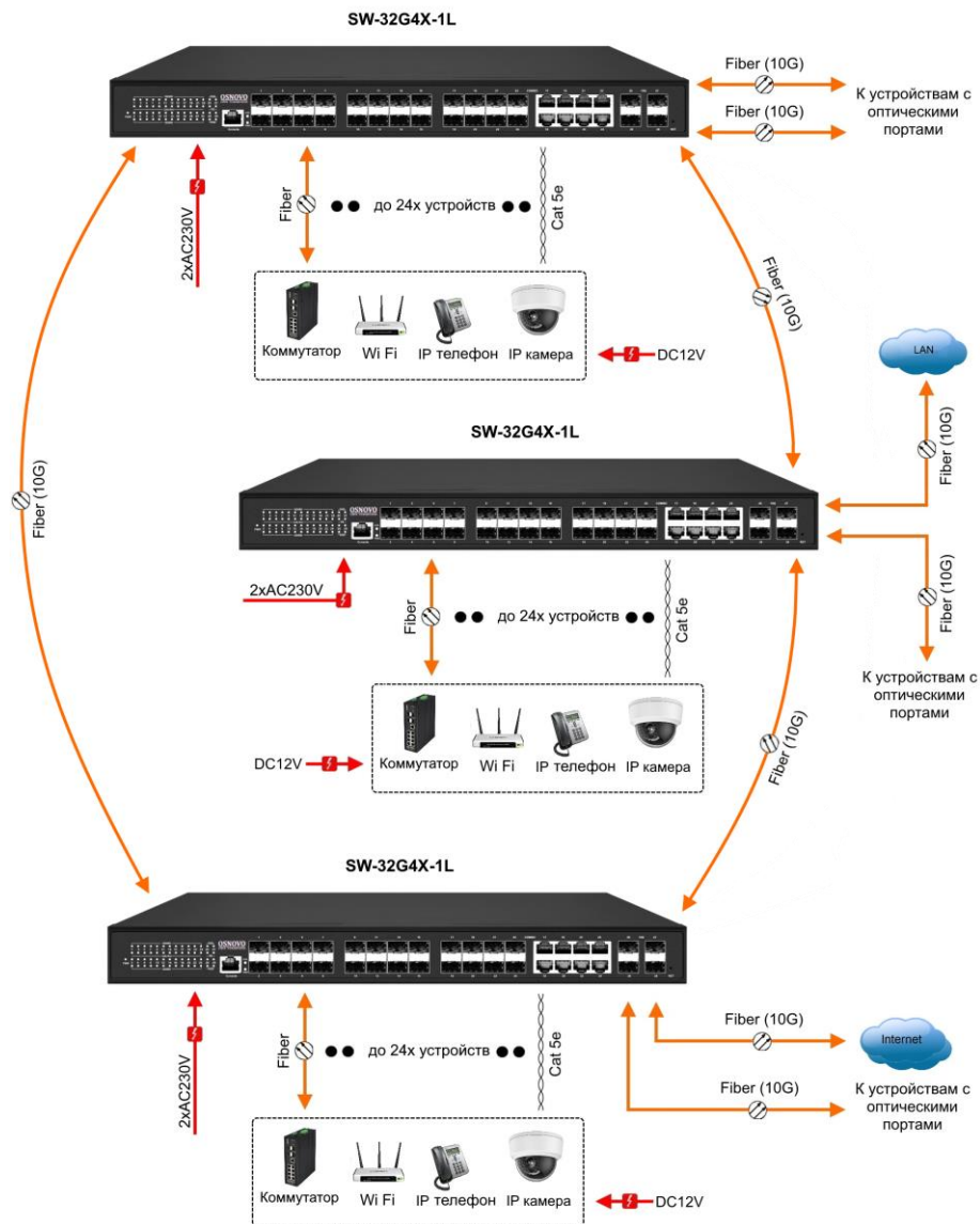
Рис.4 Кольцевая схема подключения коммутатора SW-32G4X-1L
