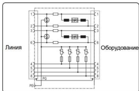
Рис.3 Внешний вид и электрическая схема SP-IP/100PS.
