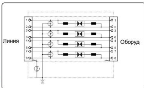
Рис.1 Внешний вид и электрическая схема SP-IP/100(ver.2), SP-IP/100D
