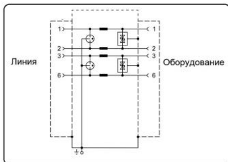
Рис.4 Внешний вид и электрическая схема SP-IP4/100
