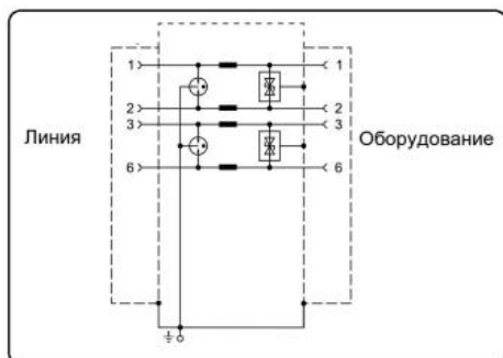
Рис.5 Внешний вид и электрическая схема SP-IP8/100(ver.2)
