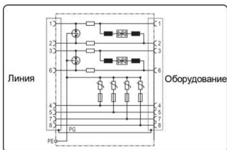
Рис.2 Внешний вид и электрическая схема SP-IP/100PD.
