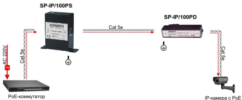
Рис. 11 Схема подключения SP-IP/100PD, SP-IP/100PS
