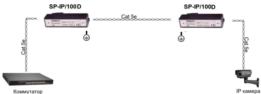
Рис. 10 Схема подключения SP-IP/100(ver2) , SP-IP/100D , на примере SP-IP/100D .
