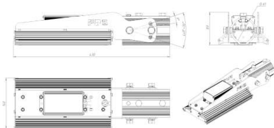
Рис. 1. Габаритные размеры светильника FOS Road R-60
