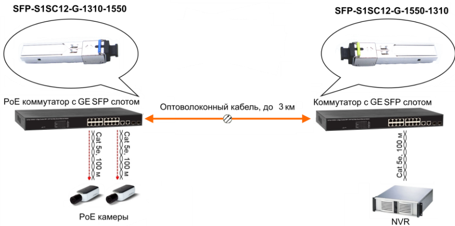
Рис.4 Типовая схема подключения SFP модулей SFP-S1SC12-G-1310-1550, SFP-S1SC12-G-1550-1310
