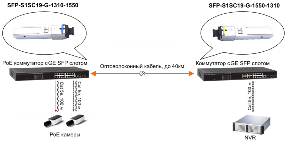
Рис.6 Типовая схема подключения SFP модулей SFP-S1SC19-G-1310-1550, SFP-S1SC19-G-1550-1310
