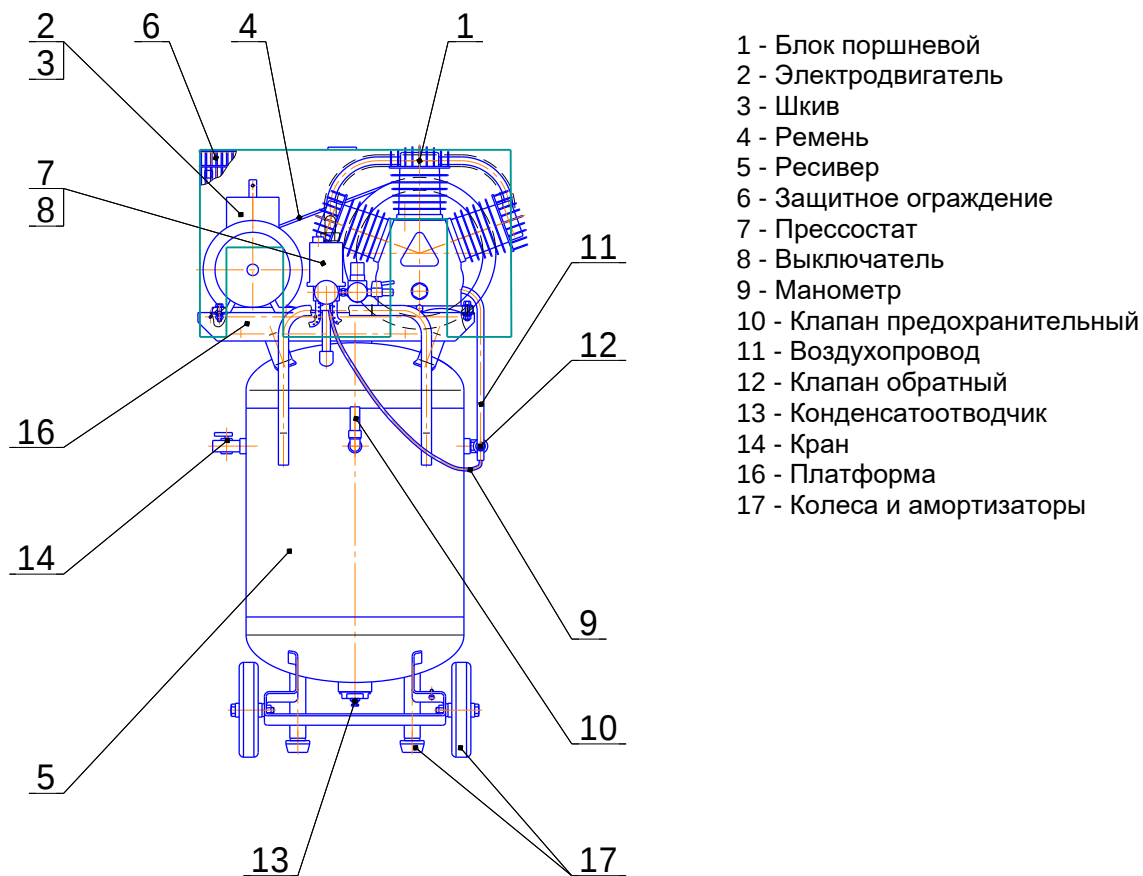
Рисунок 7 - Общий вид компрессора СБ4/С-100.LB40В
