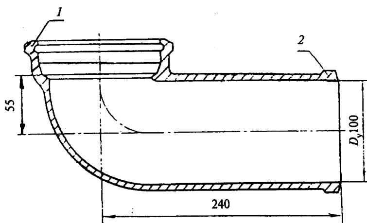
1 — раструб типа IV; 2 — хвостовик Рисунок 11
