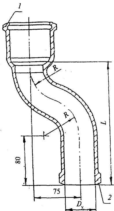
1 — раструб типа I; 2 — хвостовик Рисунок 14
