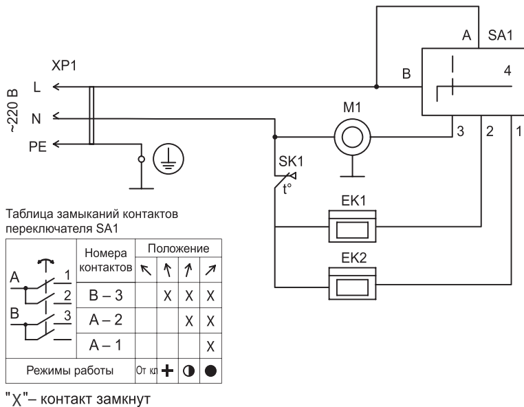
Схема электрическая ТПК-2,ТПК-3
