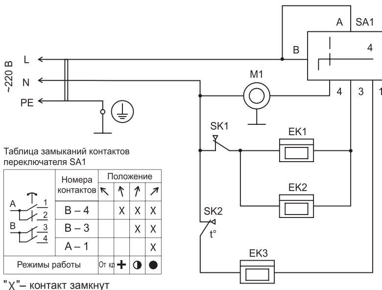
Схема электрическая ТПК-5
