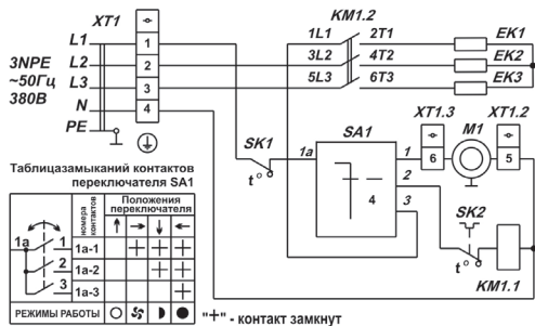
Схема электрическая принципиальная ТПП-6, ТПП9
