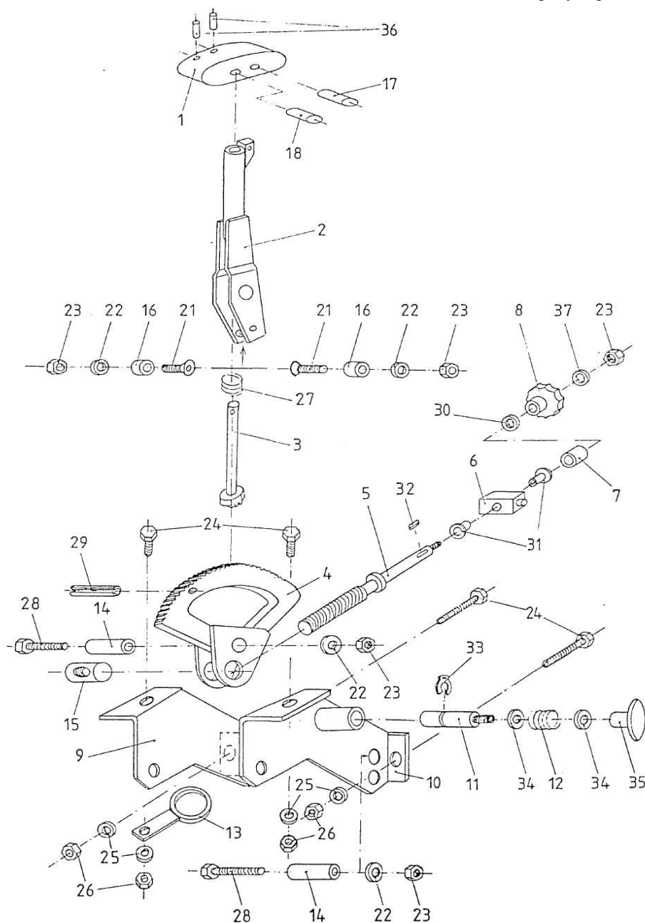
665.10.00: Перечень деталей механизма регулирования
