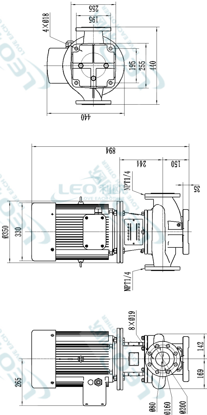
LPP80-28-11/2安装尺寸图
