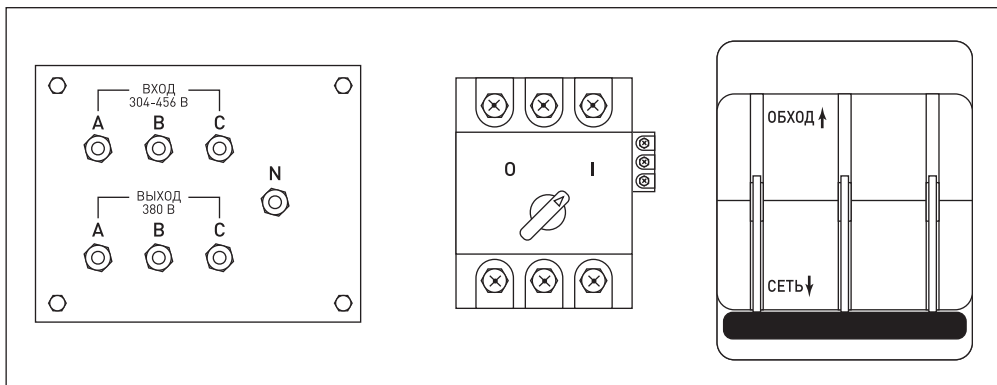
1. Клеммная колодка
