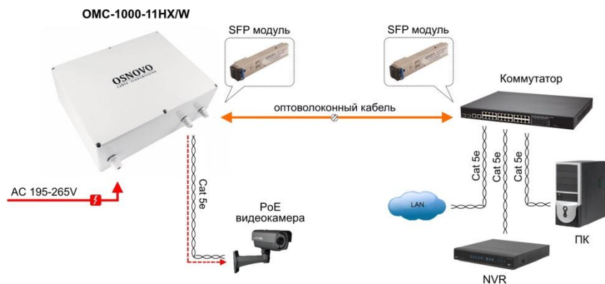
Рис.6 Типовая схема подключения медиаконвертера OMC-1000-11HX/W
