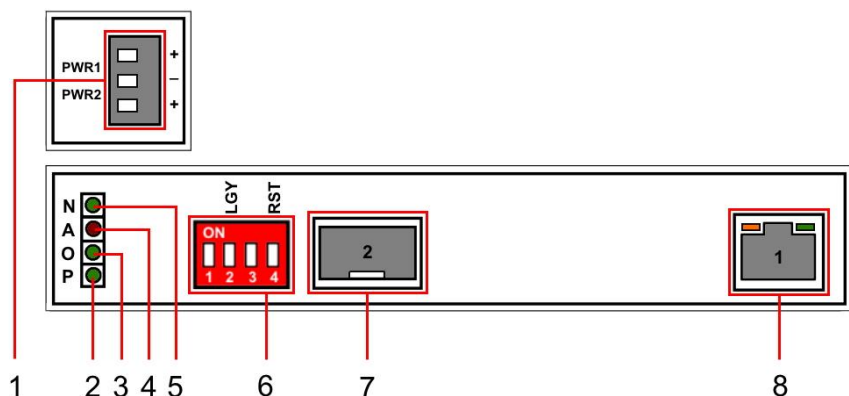
Рис. 3 Медиаконвертер ОМС-1000-11НХ/W, разъемы и индикаторы
