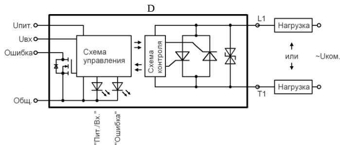
D – реле
