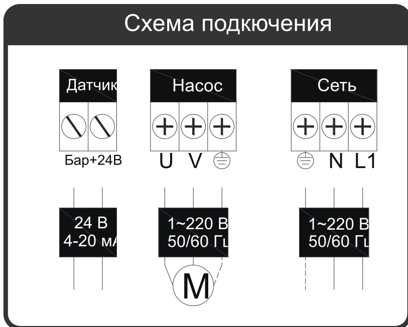
Схема подключения к однофазной сети питания
