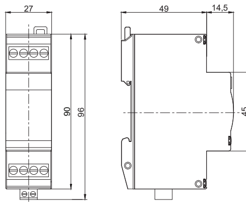
Габаритные размеры
