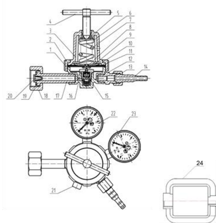
Рис. 1. Редуктор баллонный одноступенчатый
