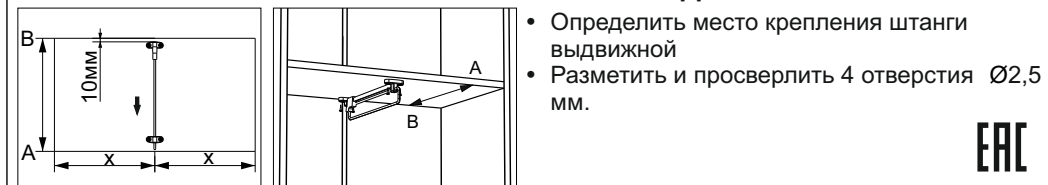
Схема Г. Установка штанги выдвижной
