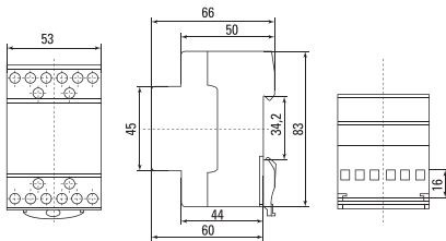
Рис.3 Габаритные размеры трансформаторов 30ВА
