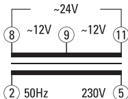
Рис. 1 Принципиальная схема звонкового трансформатора
