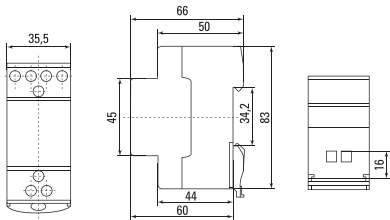
Рис. 2 Габаритные размеры трансформаторов 15ВА
