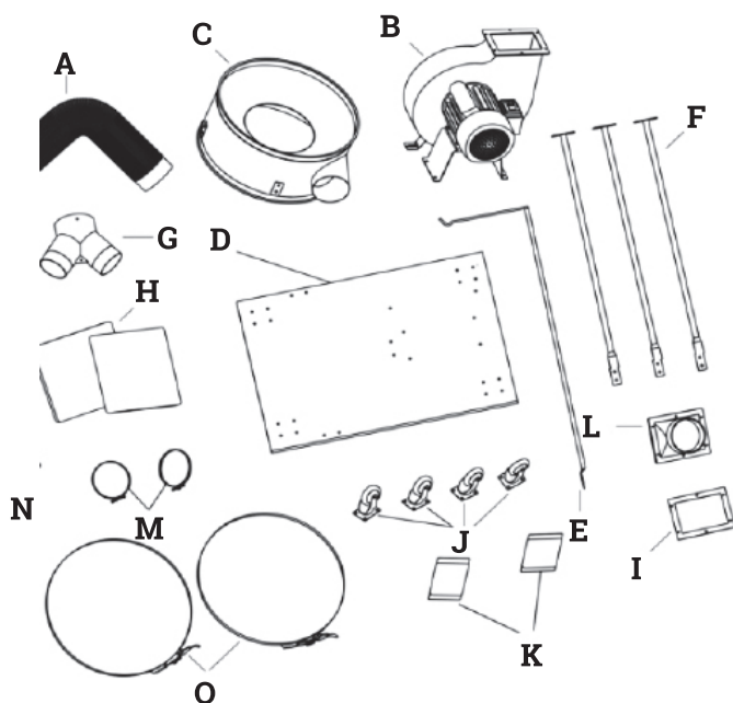
Рис. 1 Распаковать коробку. Проверить прибор, сверить со списком деталей
