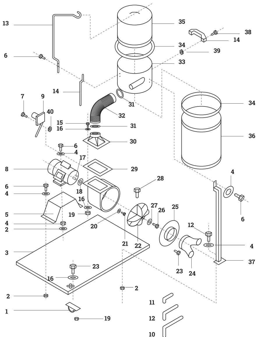
Рис. 2 Схема расположения деталей стружкоотсоса
