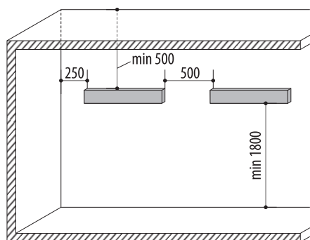
Рисунок 4. Минимальные расстояния (мм) от обогревателя до других поверхностей.
