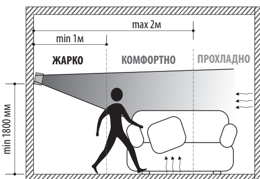
Рисунок 5. Распределение тепла в объеме помещения
