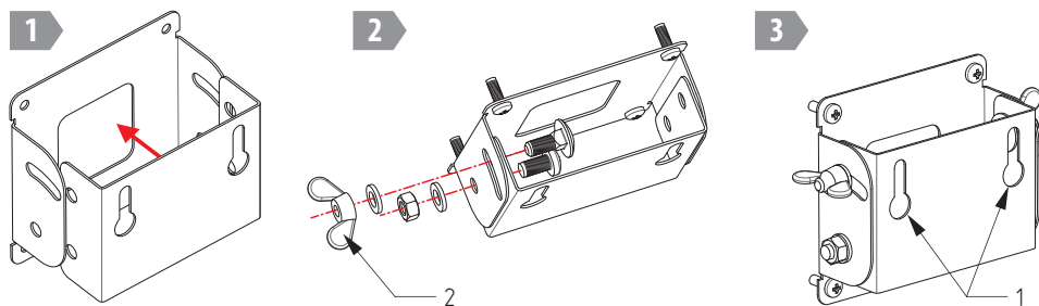
Рисунок 2. Схема сборки стенового кронштейна.
