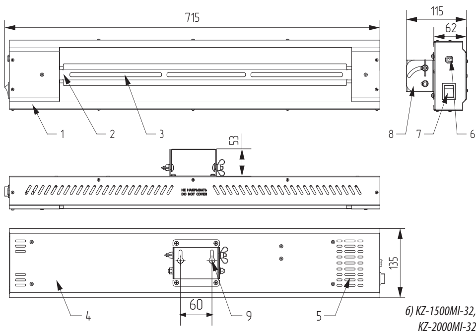
Рисунок 1. Габаритный чертёж и элементы конструкции электрического обогревателя
