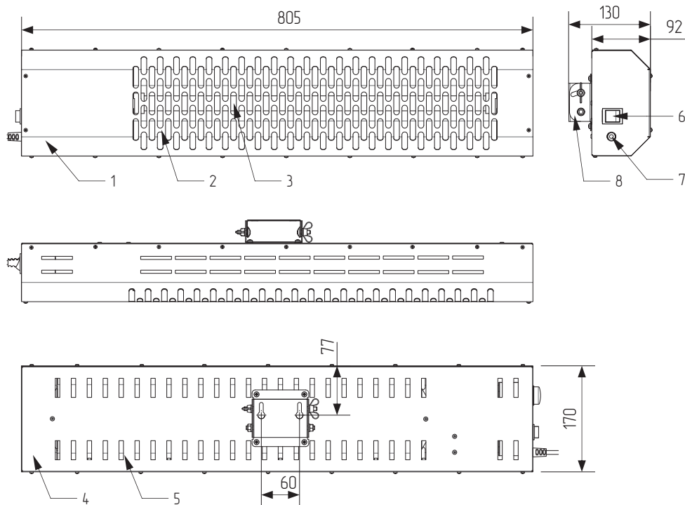
Рисунок 2. Габаритный чертёж и элементы конструкции электрического обогревателя KZ-1500MI-INOX, KZ-2000MI-INOX.
