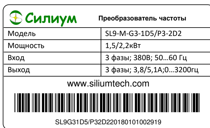
Рис 2-1 Обозначение и этикетка
