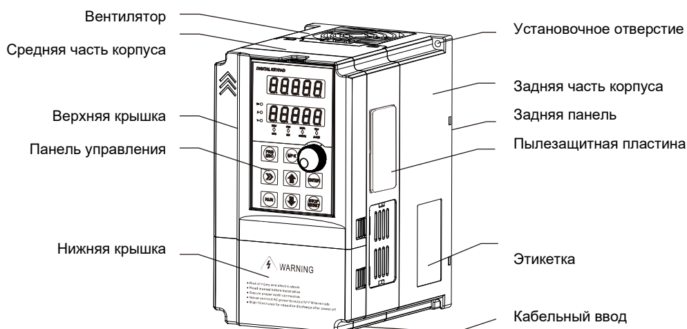
Рис 2-2 Внешний вид
