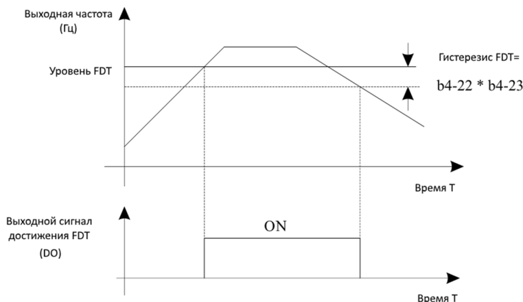
Рис. 5-14 уровень FDT
