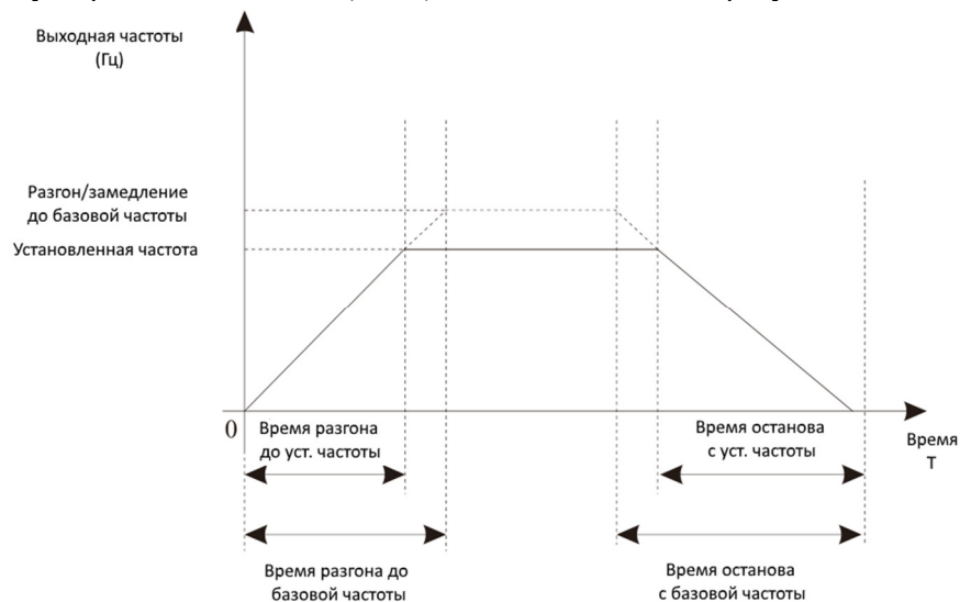
Рис. 5-3 Время разгона/торможения
