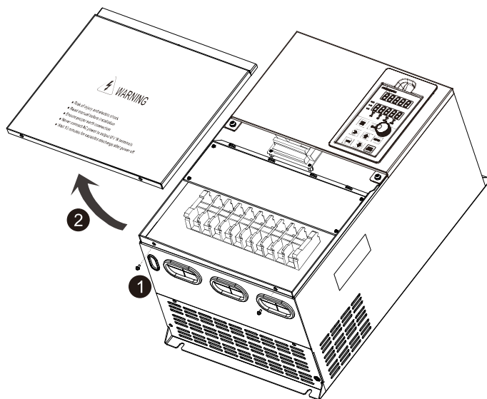
Рис. 3-6 SL9 в металлическом корпусе
