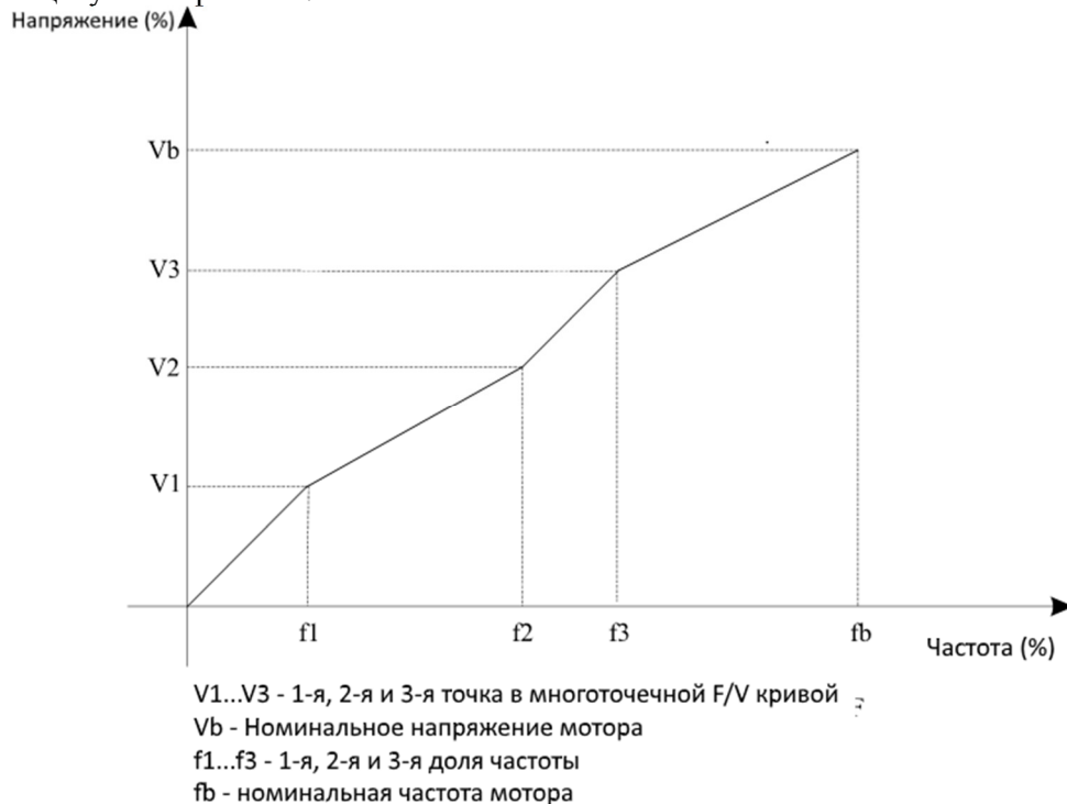
Диаграмма 5-31 Настройка многоточечной кривой V / F
