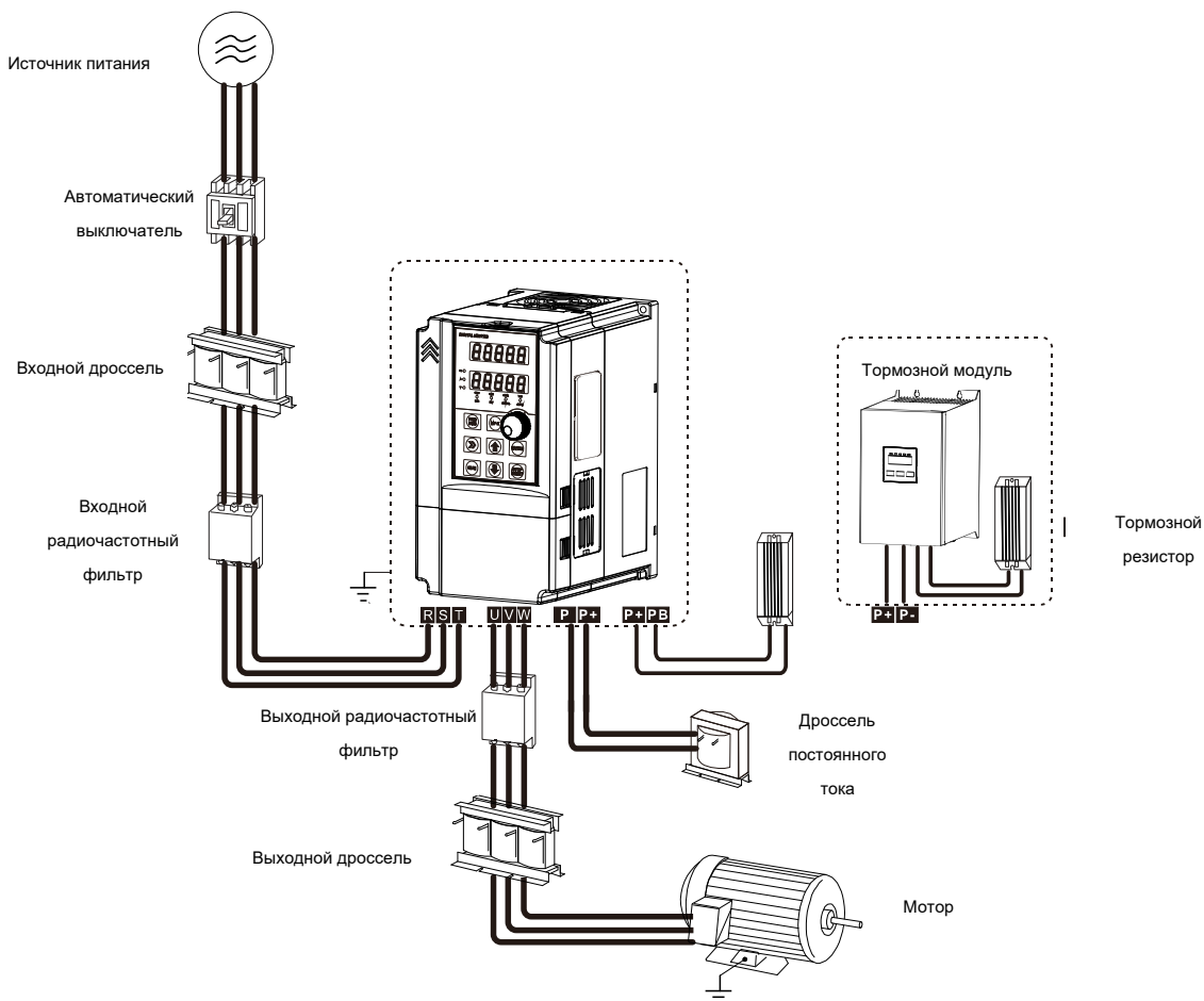
Рис. 3-2 Периферийное оборудование
