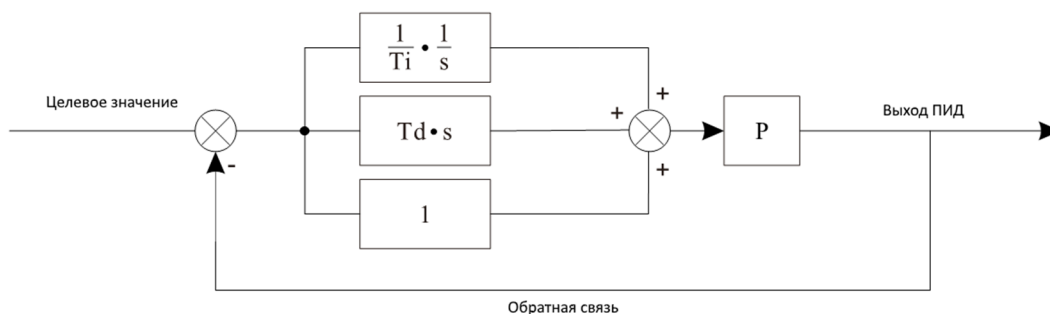
Рис. 5-25 Блок-схема ПИД-регулирования.
