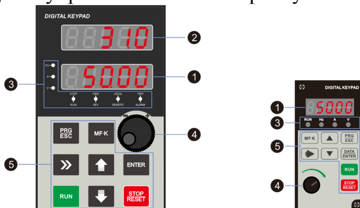
Рис. 4-1 Панель управления
