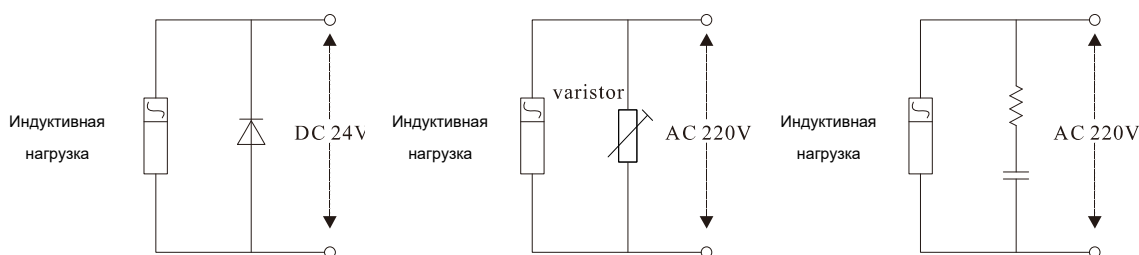
Рис. 3-10 Пример применения индуктивного ограничителя перенапряжения
