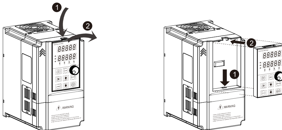
Рис. 3-3 Удаление панели управления (клавиатуры) Рис. 3-4 Установка панели управления (клавиатуры)
