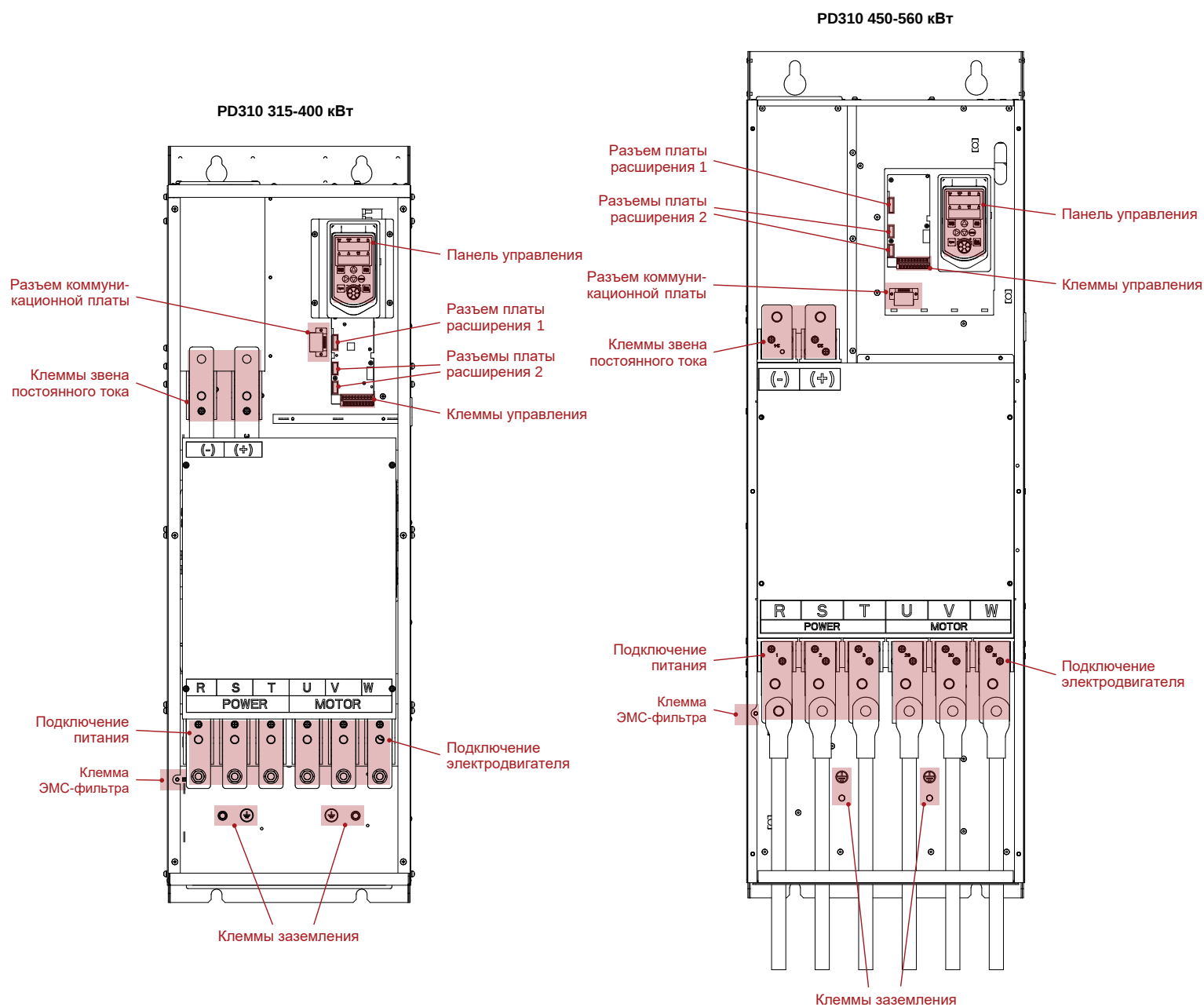
Рисунок 4-4 Расположение клемм преобразователей частоты 315-560 кВт
