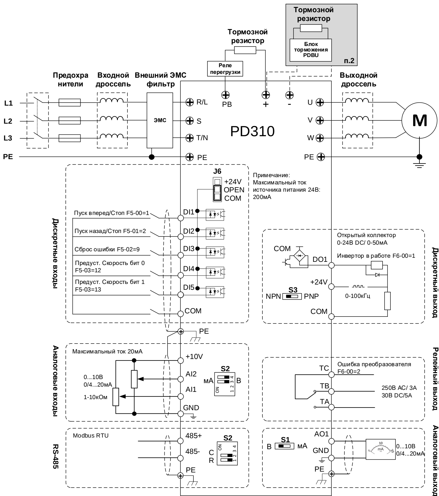
Рисунок 4-11 Типовая схема подключения
