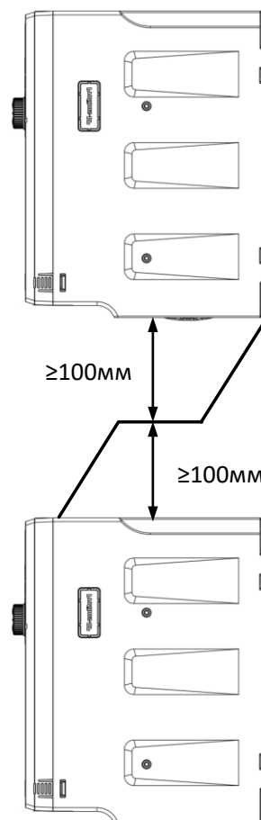
Дефлектор воздушного потока при монтаже преобразователей друг над другом
