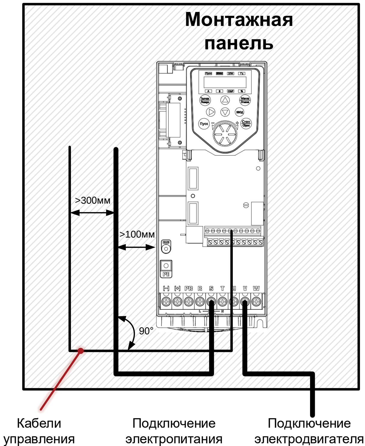
Рисунок 4-8 Схема прокладки силовых и сигнальных кабелей
