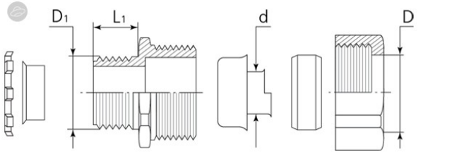
Приложение 2 – Последовательность сборки вводного узла оповещателей
