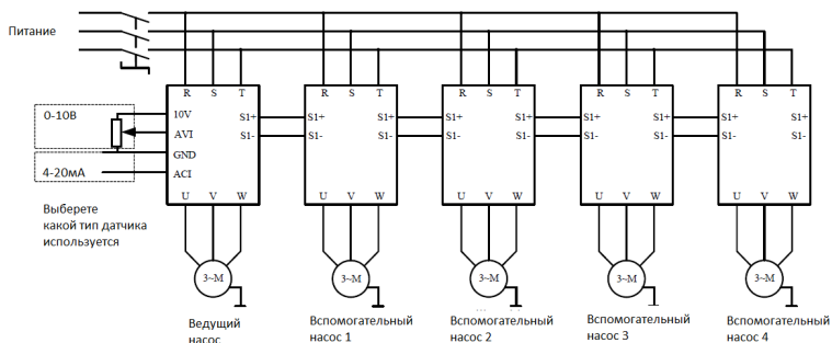
7 Подключение нескольких насосов мастер/слейв (клеммы)
