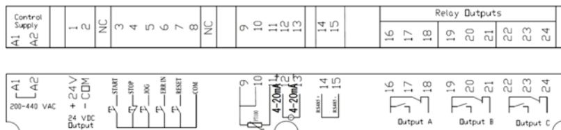
Рис 4.6 Клеммы цепей управления SL-IB3.
