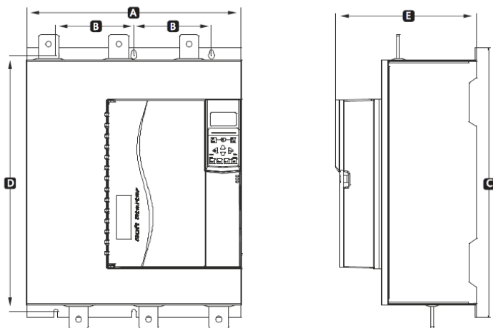
3 Габаритные размеры УПП 132-500кВт
