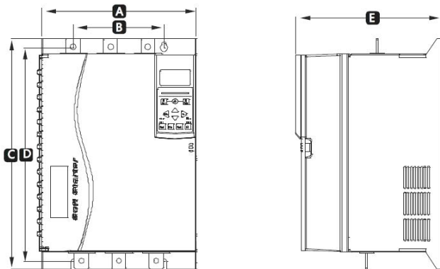
2 Габаритные размеры УПП 75-115кВт
