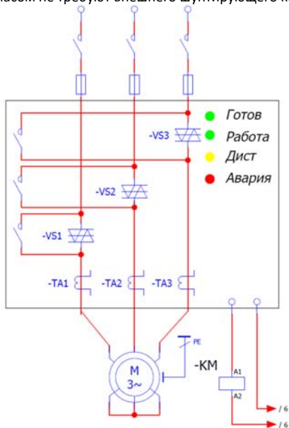
Рис. 4.4 Схема подключения SL-IB3 при работе в «звезде».
