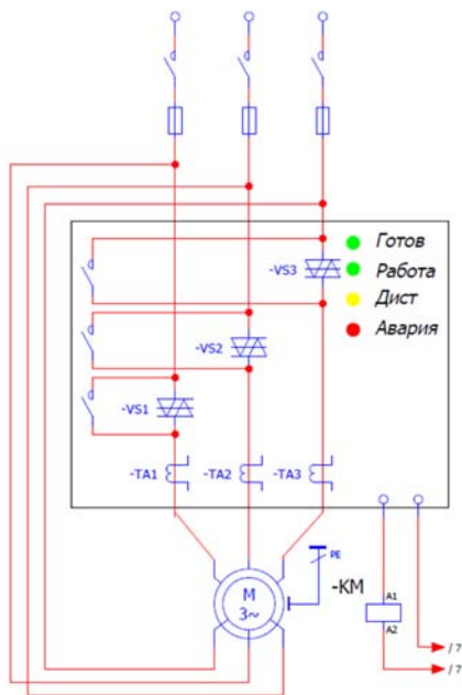
Рис. 4.4 Схема подключения SL-IB3 при работе в «звезде».
