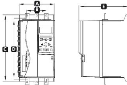
1 Габаритные размеры УПП 11-55кВт
