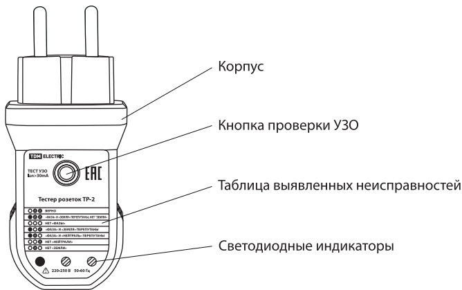
Рисунок 1. Внешний вид и конструкция тестера
