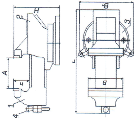
1 - губка подвижная; 2 - корпус; 3 - плита поворотная; 4 - рукоятка Рисунок
