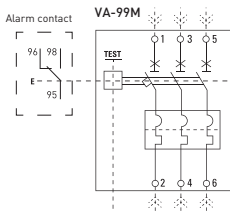
Fig. 1 - Wiring diagram
