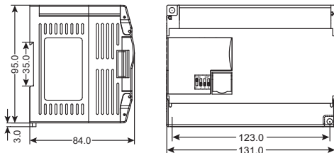
Рис. 2 - Габаритные размеры модулей EREMF-D-40X, EREMF-D-36Y-R, EREMF-D-36Y-N, EREMF-D-20X20Y-R, EREMF-D-20X20Y-N
