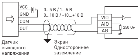
Рис. 4в - Подключение аналоговых входов (входной сигнал – напряжение)
