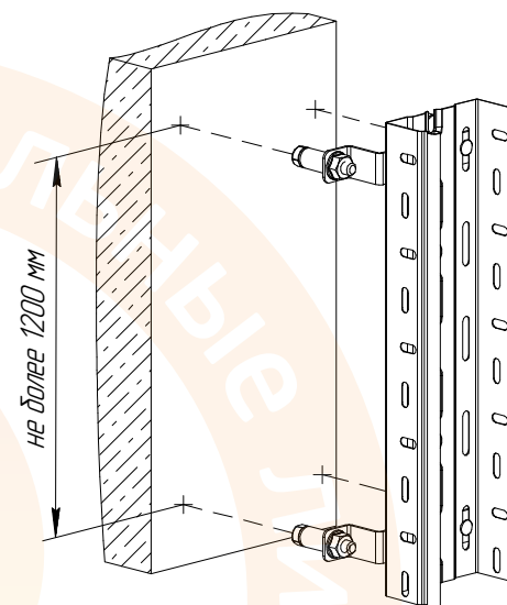
Вертикальная прокладка
