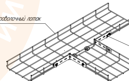
п3 Пластина соединительная для проволочного лотка Промрукав Арт. PR08.2282
