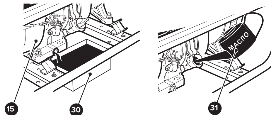
Рисунок 4 — Проверка уровня масла в картере двигателя
