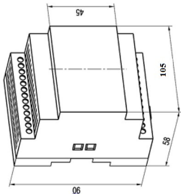
Рис1. Размеры корпуса.
