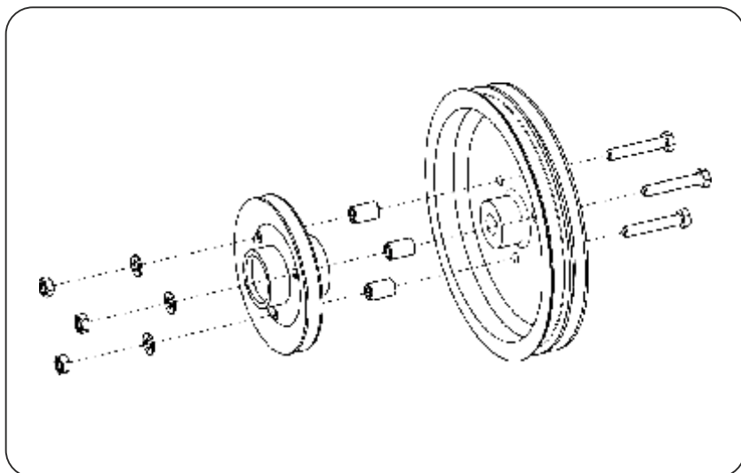
Рис.3 - Установка ведущего шкива (для МБ «Каскад» и пр.)
