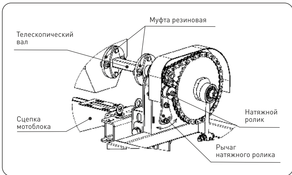
Рис.6 - Схема присоединения картофелевыкапывателя к мотоблоку (02.01.02, 02.01.04) .
