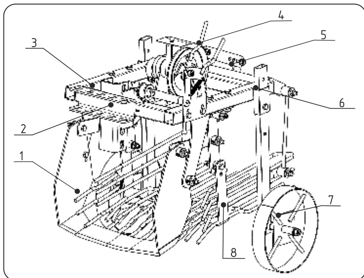
Рис.1 Общий вид (02.01.01, 02.01.03)
