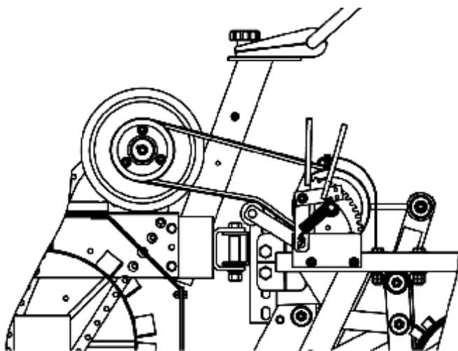
Рис.5 - Установка приводного ремня.
