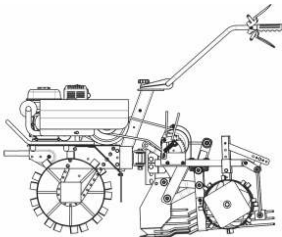
Рис.7 - Мотоблок с картофелевыкапывателем.
