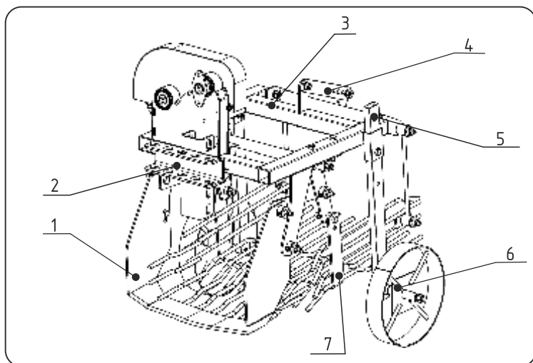
Рис.2 Общий вид (02.01.02, 02.01.04)
