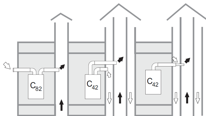
Рис. 6. Примеры систем дымоудаления собранных с помощью отдельных труб. Белой стрелкой обозначен приток воздуха, чёрной стрелкой поток продуктов сгорания.
