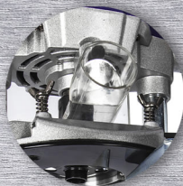
ПАТРУБОК ДЛЯ ПОДКЛЮЧЕНИЯ К ПЫЛЕСОСУ
