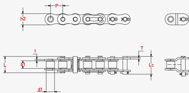
Однорядные цепи
