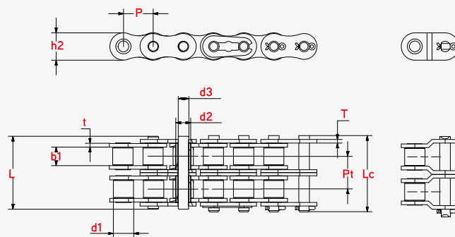
Двухрядные цепи
