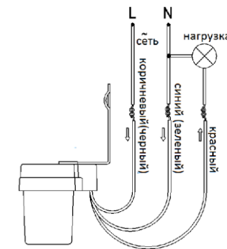
Рис. 2 Схема электропитания
