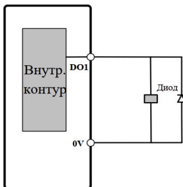
Рисунок 2-19 Подключение цифрового выхода
