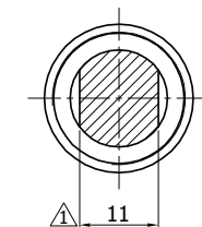
Разрез "А-А"
