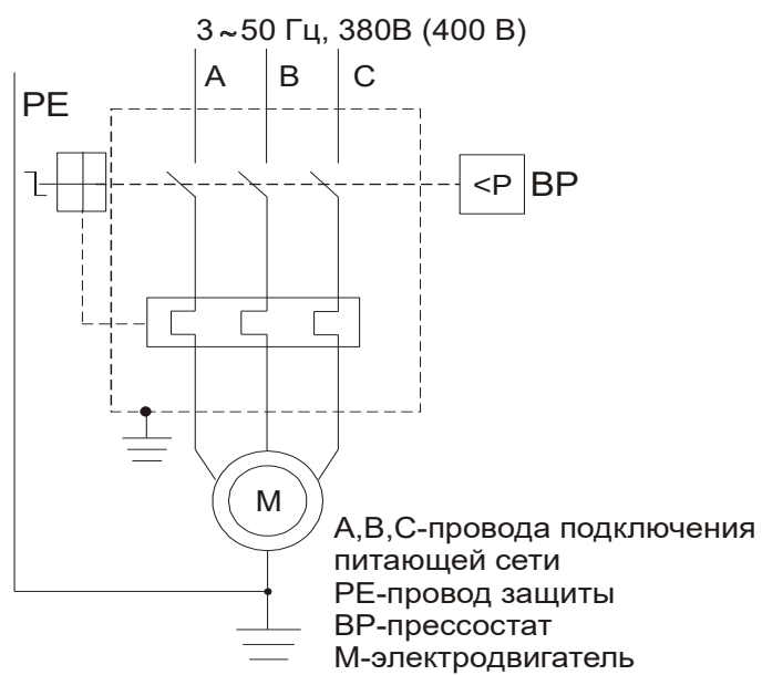
Рисунок А.1 - Схема электрическая принципиальная компрессоров СБ4/С-50.ЛВ24, СБ4/С-100.ЛВ24
