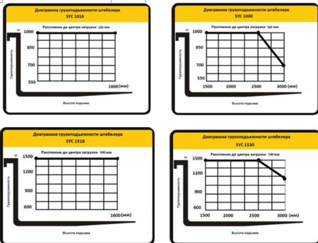
Рисунок. 3. Диаграмма грузоподъемности штабелера.
