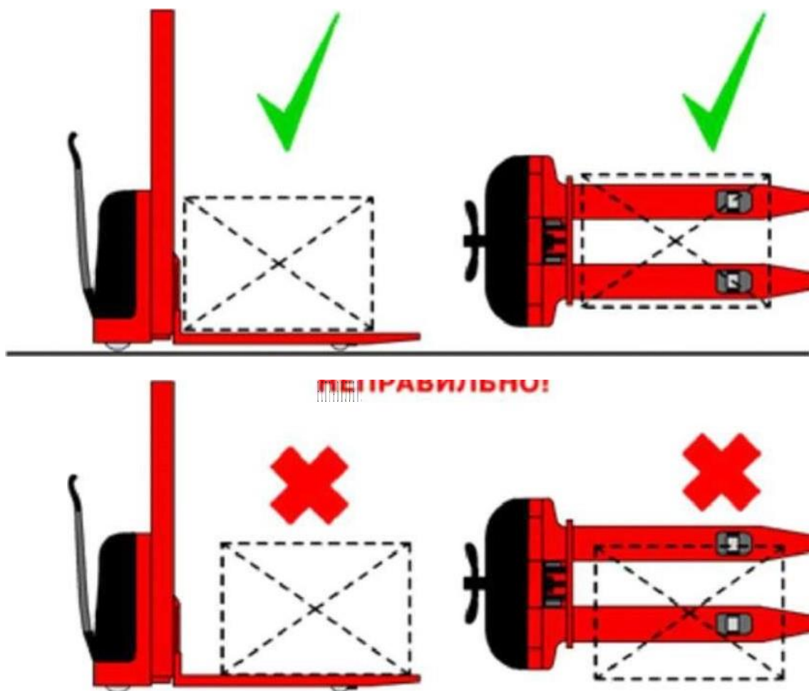
Рисунок 4. Схема расположения груза на вилках
