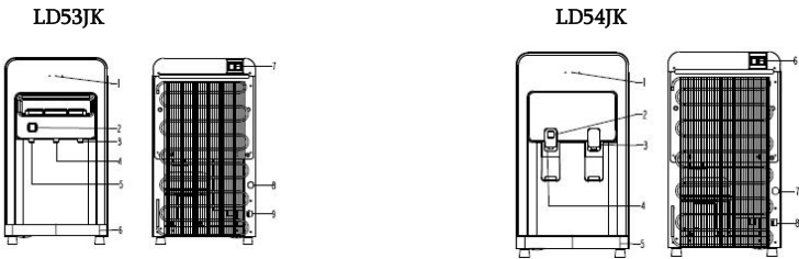
Рис.1 Наименование компонентов диспенсера
