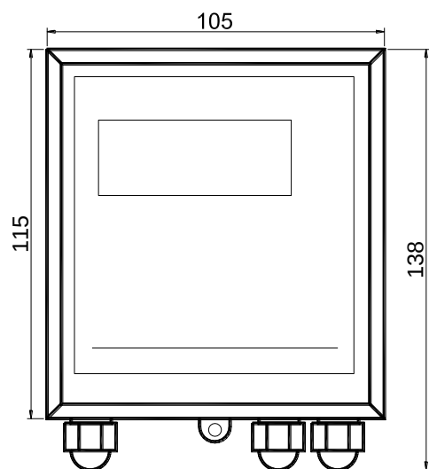
1. Эскиз корпуса настенного крепления Н1
