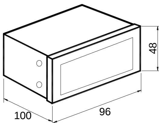
2. Эскиз корпуса щитового крепления Щ2
