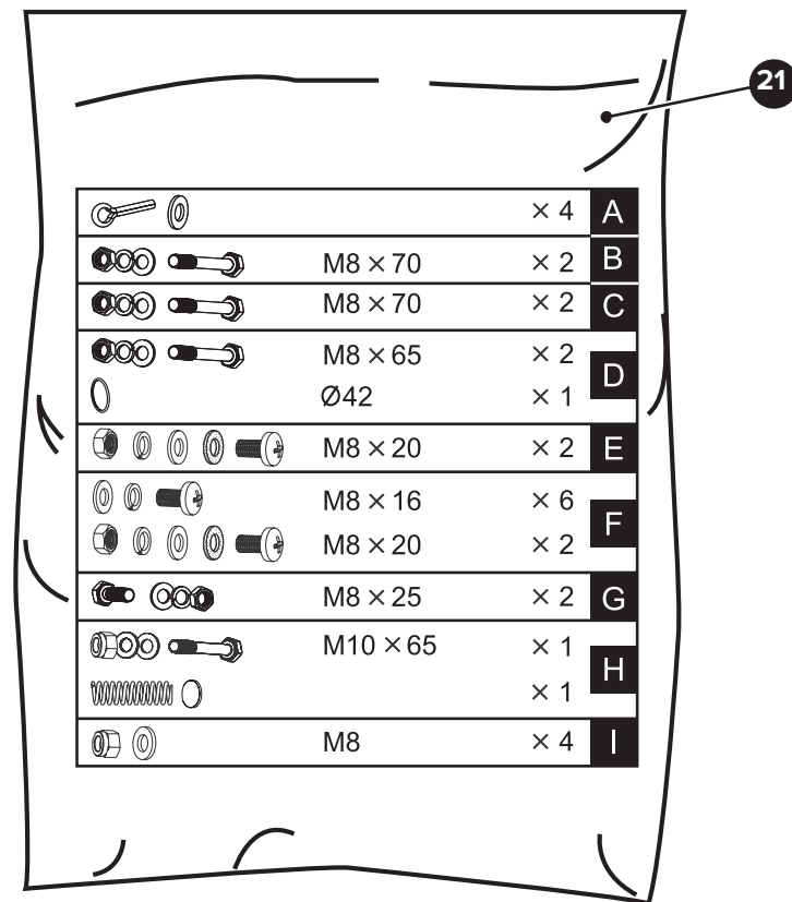
21. Мешок с 9 пакетами крепежных изделий (пакеты A, B, C, D, E, F, G, H, I). Состав пакетов с крепежными изделиями
