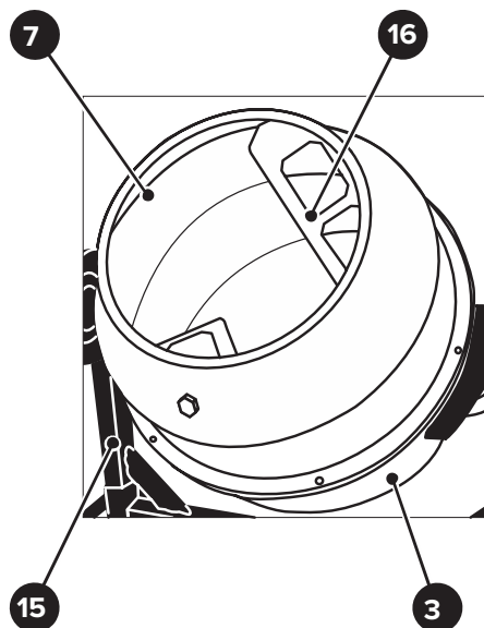
Рисунок 3 — Шнеки для замешивания раствора в барабане бетоносмесителя
