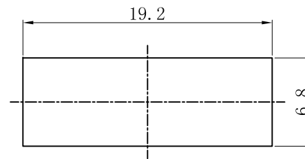
安装面板尺寸 PANEL CUT-OUT
