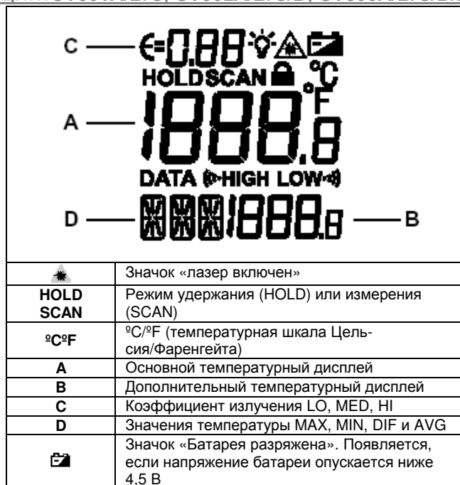
Рисунок 3. Дисплей термометра
