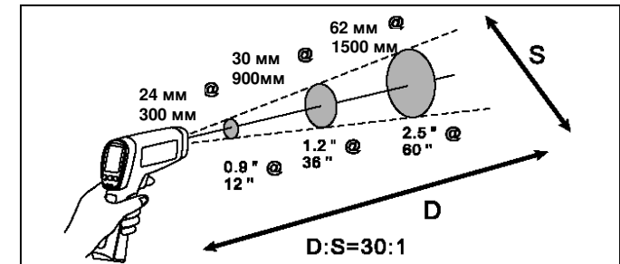
Рисунок 6. Расстояние и размер пятна
